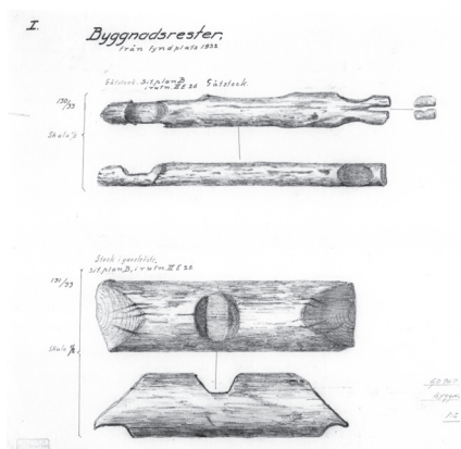
Figur 5. Exempel på delar från knuttimring som Zetterling bärgade och dokumenterade. Den övre byggnadsdelen visar en gåttstock som satt på vänster sida om en dörröppning i en gavel att döma av måtten. Gåttspåret syns som ett urtag på höger sida. Den nedre delen är den översta stocken i ett gavelröste med urtag för takåsen mitt på stockens ovansida. Byggnadsdelarna påträffades 1933. ATA, I13 I62 Go I109F.
