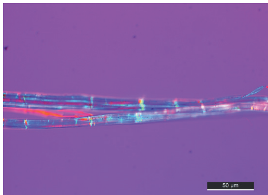
Prov M4. Polarisationsljusmikroskop (PLM) Herzog-test visar blåfärgad fiber i horisontal riktning. Foto: Jenni Suomela.
