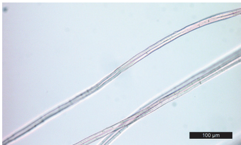
Prov M4. Transmittljusmikroskop (TLM) visar bastfibrer. Foto: Jenni Suomela.
