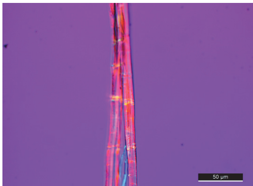
Prov M4. Polarisationsljusmikroskop (PLM) Herzog-test visar guldfärgad fiber i diagonal riktning. Foto: Jenni Suomela.
