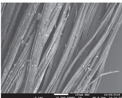
Prov M4. Svepelektronmikroskop (SEM) visar bastfibrer. Foto: Krista Vajanto.
