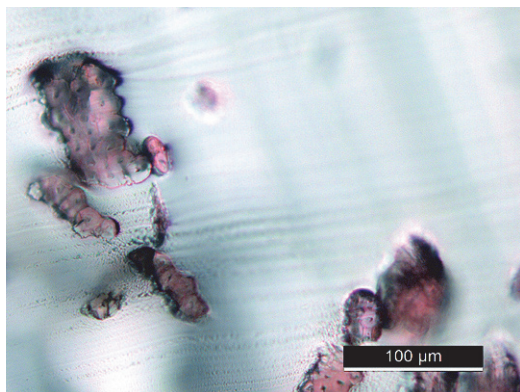
Prov M4. Cellformer i tvärsnitt i Transmittljusmikroskop (TLM). Foto: Jenni Suomela.
