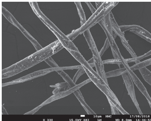
Prov M1. Svepelektronmikroskop (SEM) visar bomullsfibrer. Foto: Krista Vajanto.
