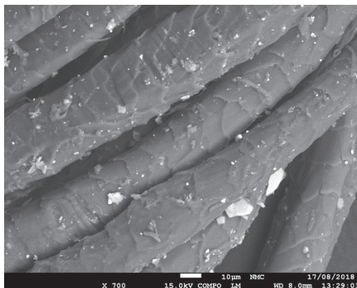
Prov M3. Svepelektronmikroskop (SEM) visar ullfibrer. Foto: Krista Vajanto.
