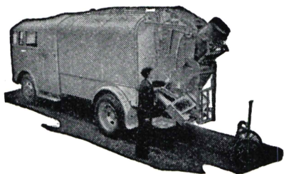
NORBA-bil typ KA med komprimering och automatisk kärlliftning och tömning. Lastar lätta sopor upp till 40 å 50 kbm.
