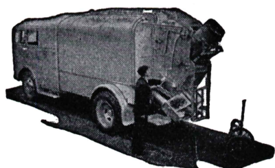
NORBA-bil typ KA med komprimering och automatisk kärlyftning och tömning. Lastar lätta sopor upp till 40 à 50 kbm.
